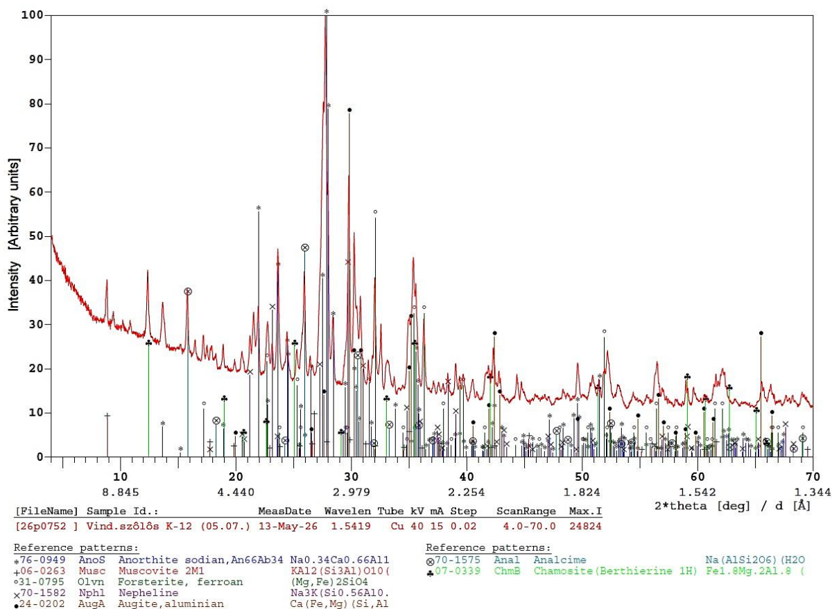
1.ábra: Vindornaszőlős (K12) jelű minta röntgendiffrakciós (XRD) felvétele
