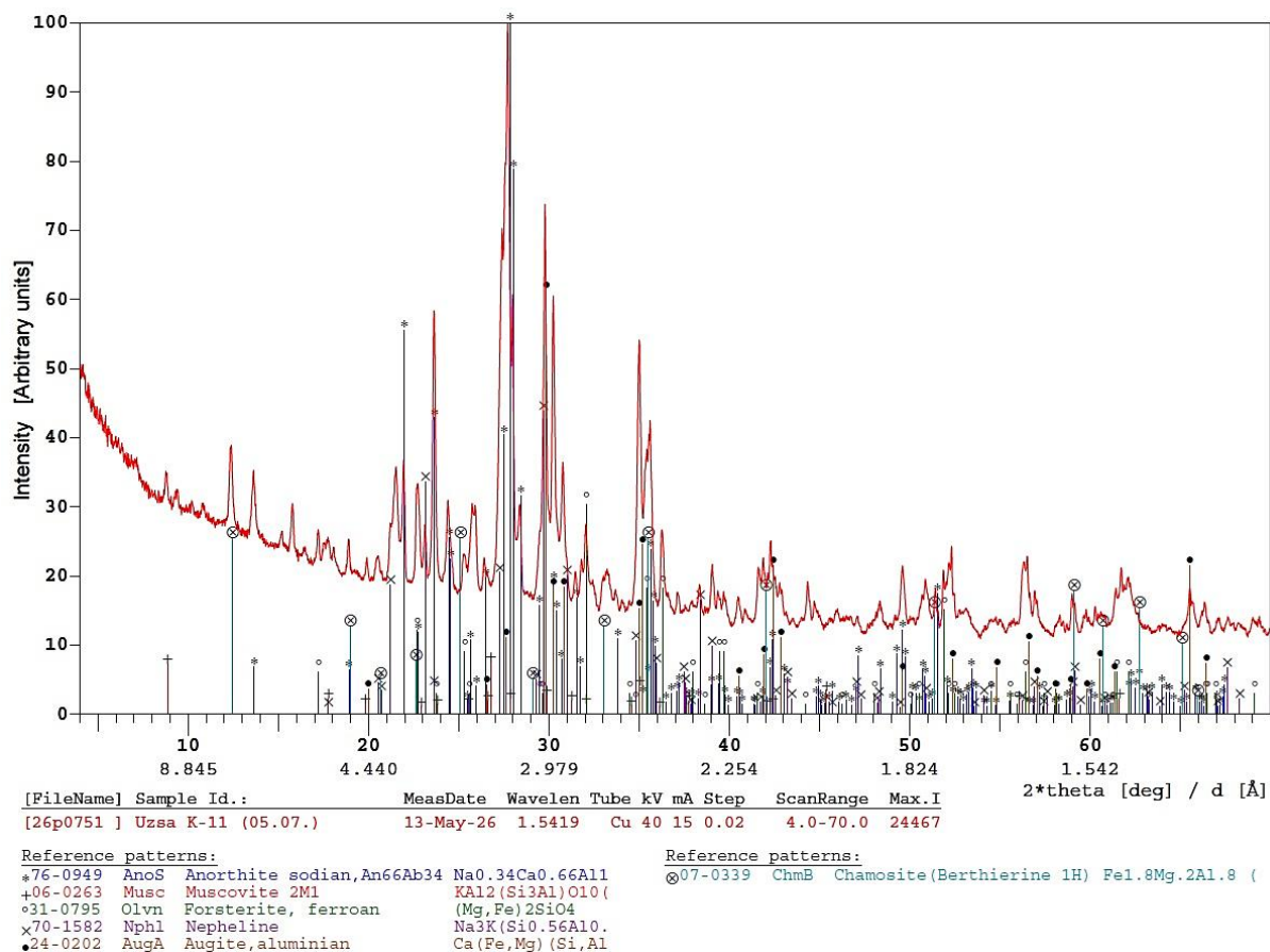
1.ábra: Uzsa (K11) jelű minta röntgendiffrakciós (XRD) felvétele
