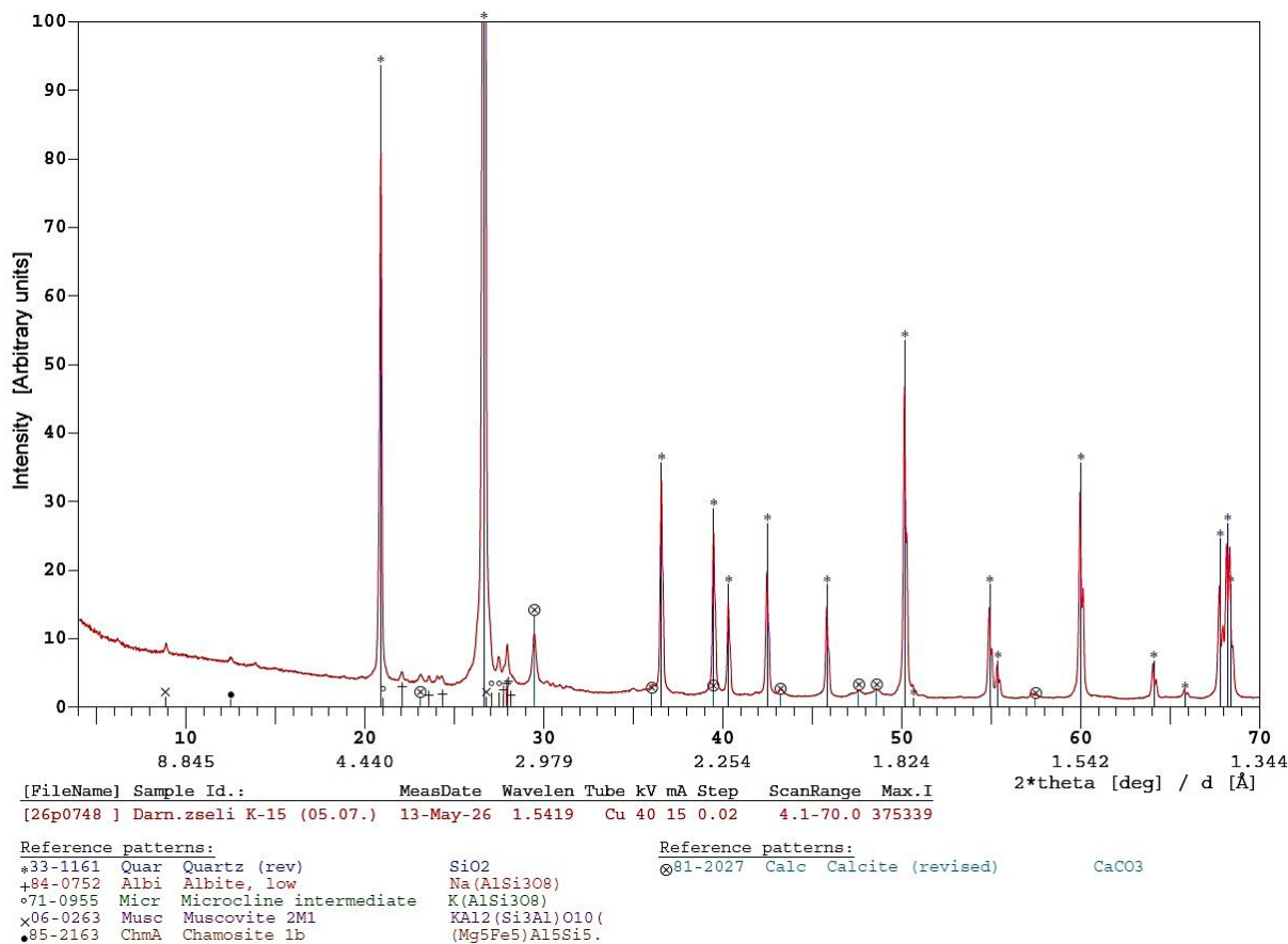
1.ábra: Darnózseli (K15) jelű minta röntgendiffrakciós (XRD) felvétele
